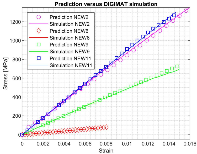
Figura 9. Comparatie între valorile reale si cele predictate pentru cele 4 specimene generate aleator
